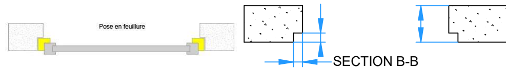
Pose Feuillure
