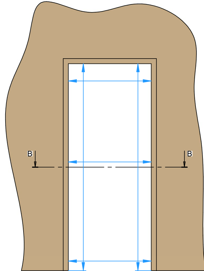
Pose Feuillure
