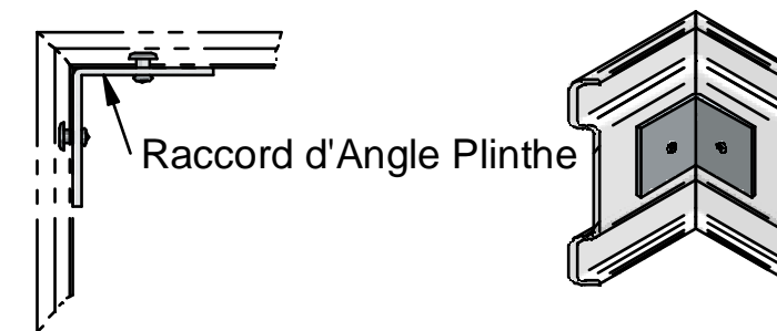
MONTAGE INTERIEUR
