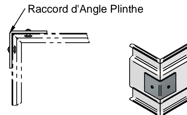
MONTAGE EXTERIEUR
