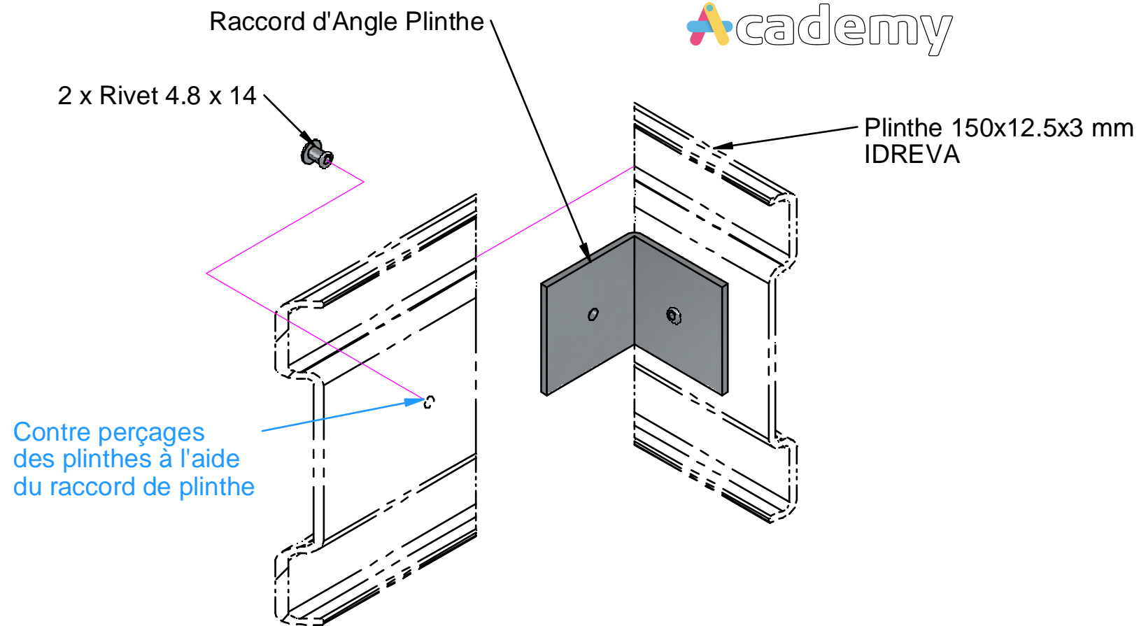
MONTAGE INTERIEUR
